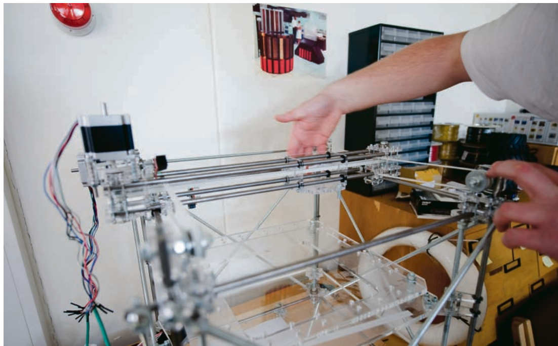
Duplikatastrofe?: Kanskje ikke visuelt imponerende, men denne dingsen kan printe ut 3D-objekter, og kanskje snart duplisere seg selv.
